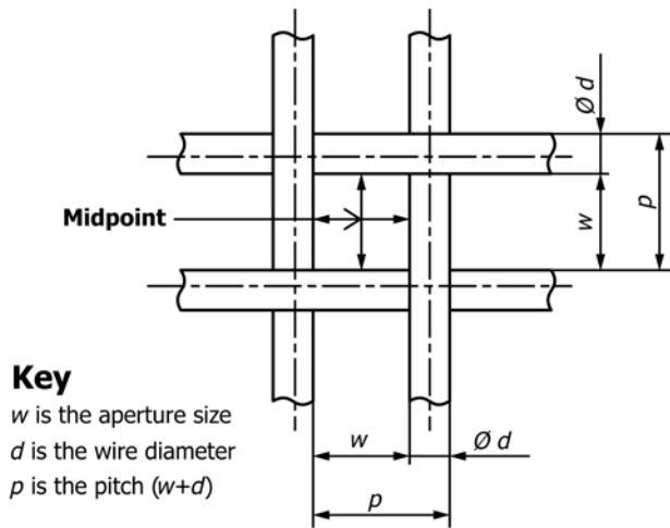
FIG. 1 Aperture Size
